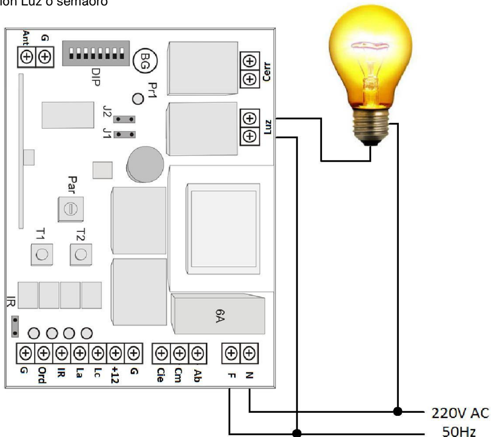
Esquema; Conexión Luz o semáforo
